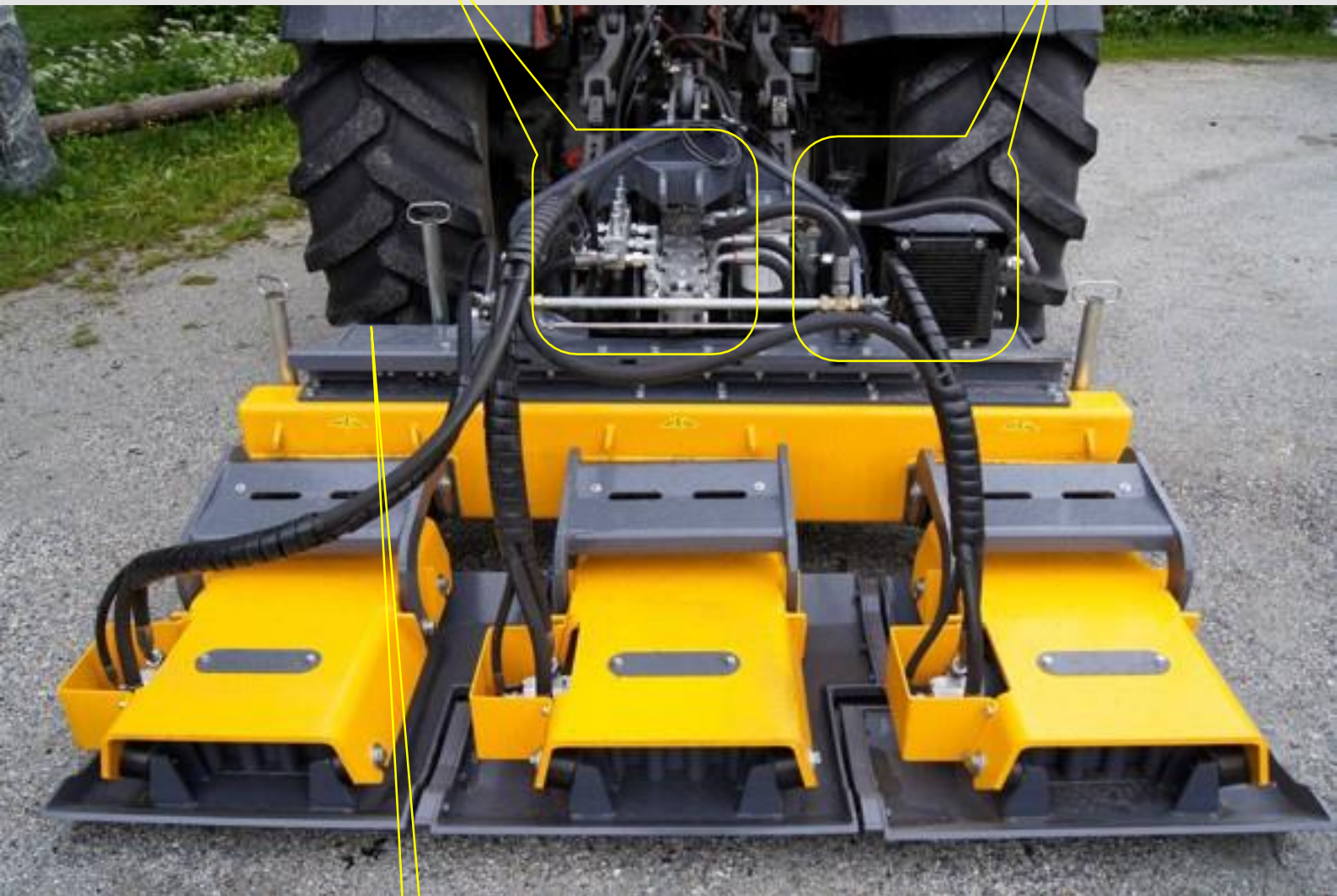
3 bombas hidráulicas impulsadas por el eje de junta universal
